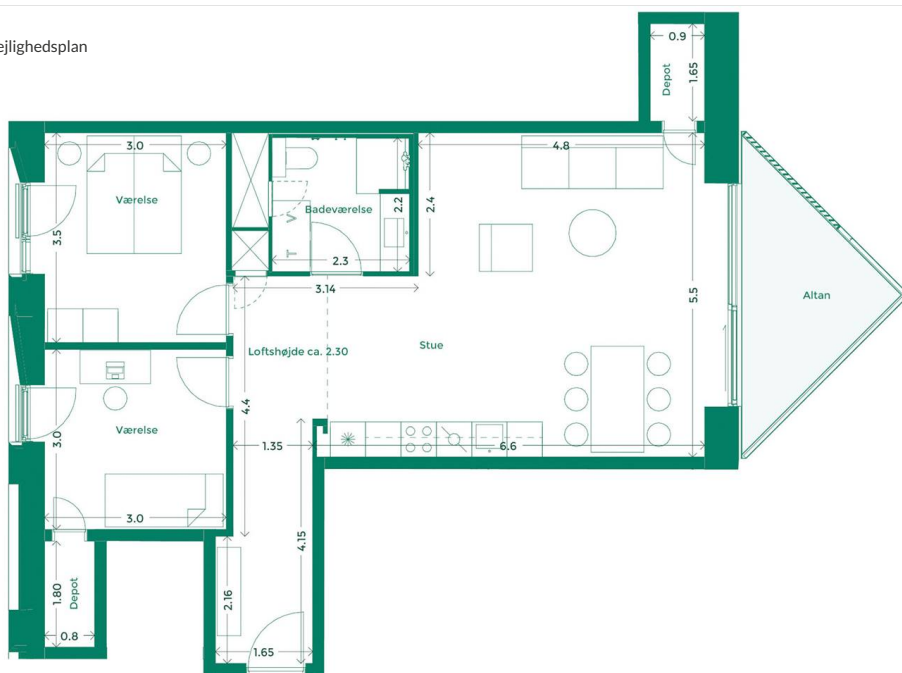
Etageplan
