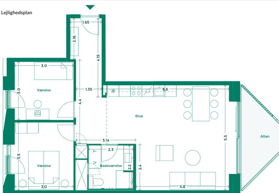
Etageplan
