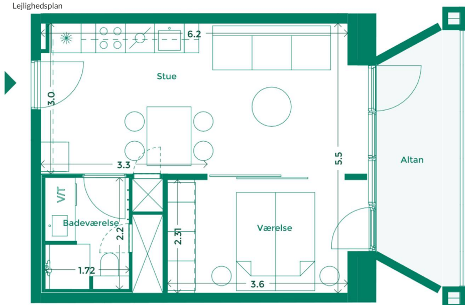
Lejlighedsplan
